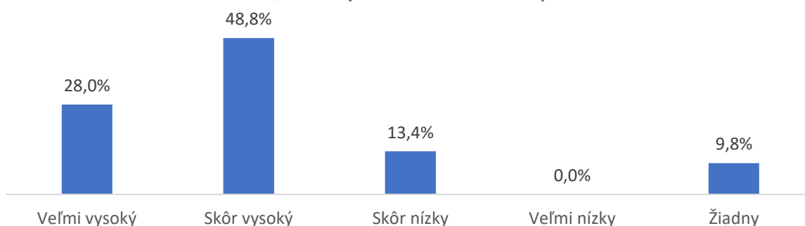
Graf č.37: Prínos služieb z externého prostredia
