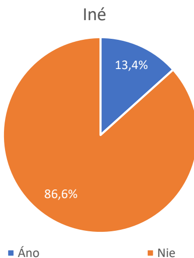
Graf č.62 Iné prekážky pre zavádzanie inovácií
