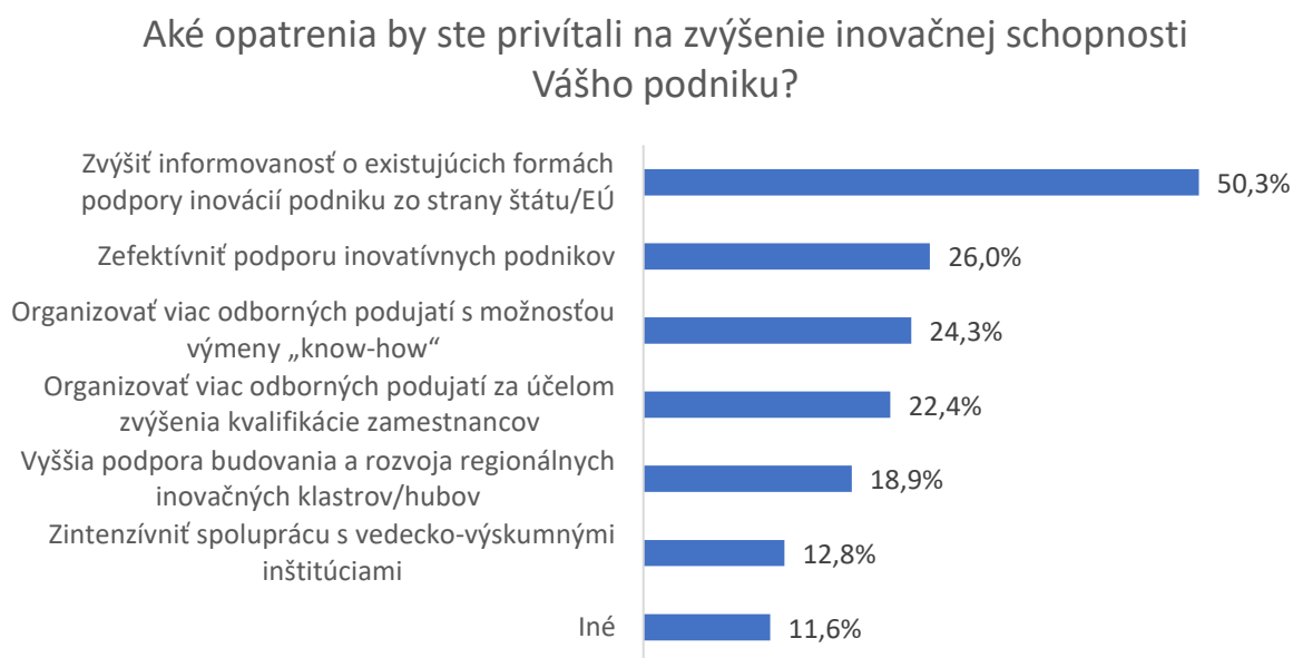
Graf č.65: Očakávané opatrenia
