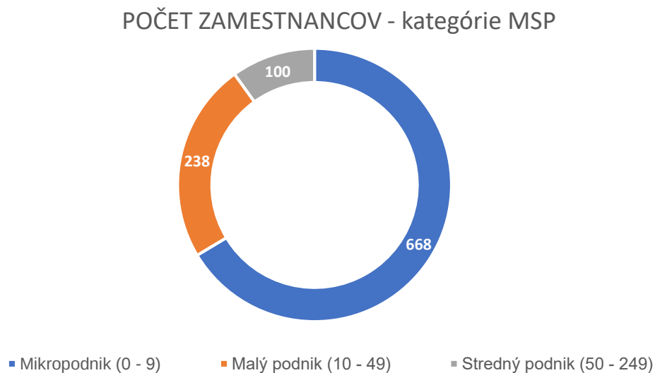
Graf č.1: Respondenti podľa počtu zamestnancov – kategórie MSP
