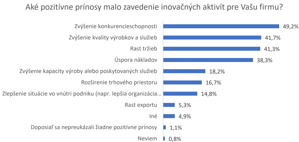
Graf č.22: Prínosy inovačných aktivít
