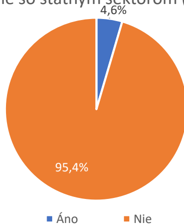
Graf č.42: Spolupráca so štátnym sektorom
