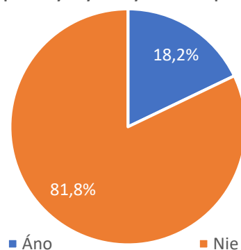
Graf č.27: Prínos: zvýšenie kapacity produkcie
