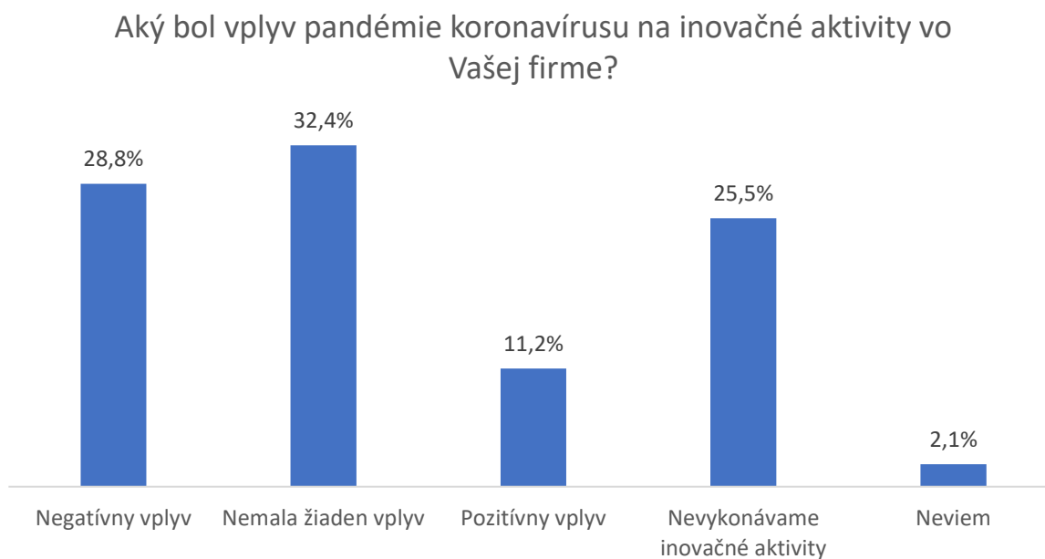
Graf č.45: Vplyv pandémie na inovácie
