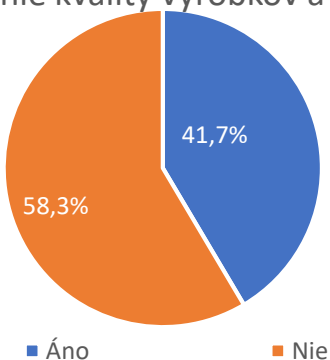
Graf č.24: Prínos: vyššia kvalita výrobkov / služieb
