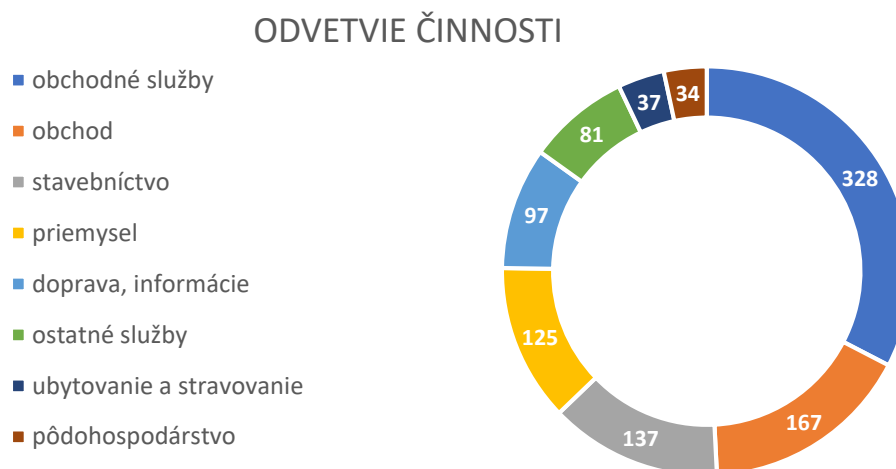
Graf č.6: Respondenti podľa odvetvia podnikateľskej činnosti
