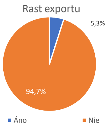
Graf č.30: Prínos: rast exportu
