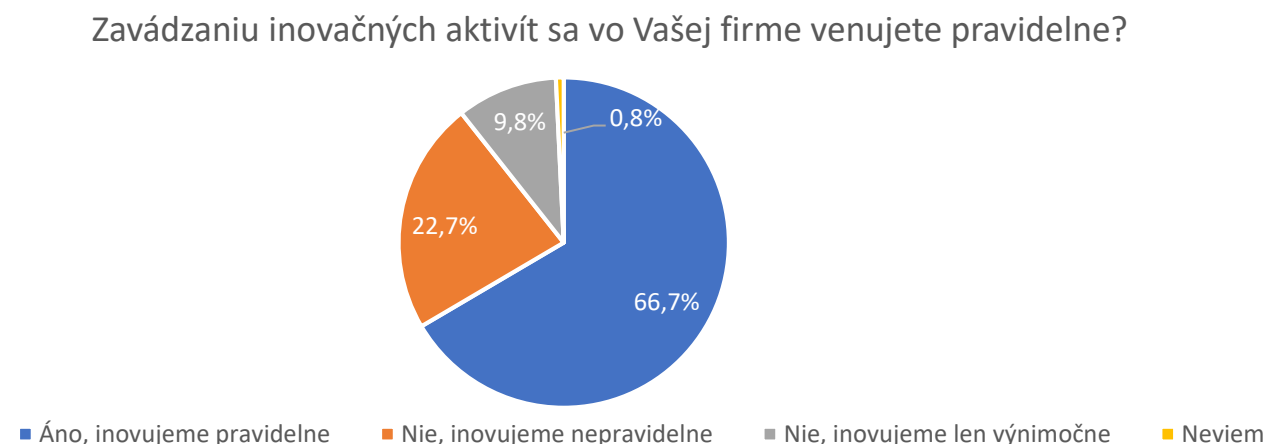
Graf č.12: Pravidelnosť inovačných aktivít
