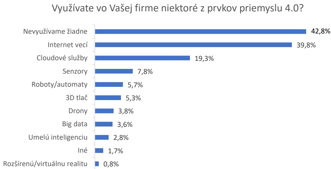
Graf č.46: Využívanie prvkov priemyslu 4.0
