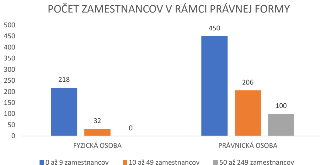
Graf č.4: Respondenti podľa počtu zamestnancov a právnej formy
