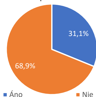
Graf č.36: Služby z externého prostredia
