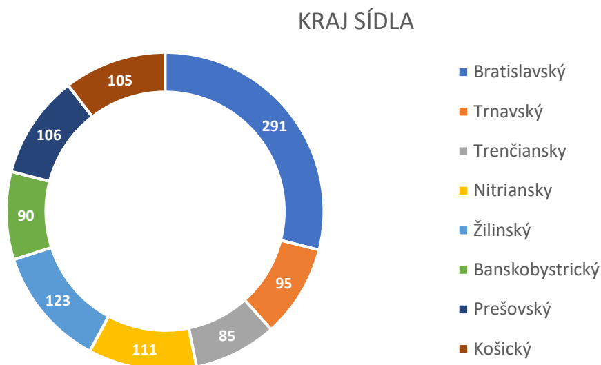
Graf č.8: Respondenti podľa kraja
