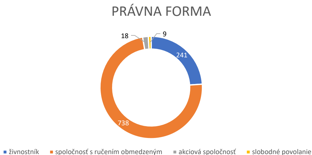
Graf č.5: Respondenti podľa konkrétnej právnej formy podnikateľského subjektu
