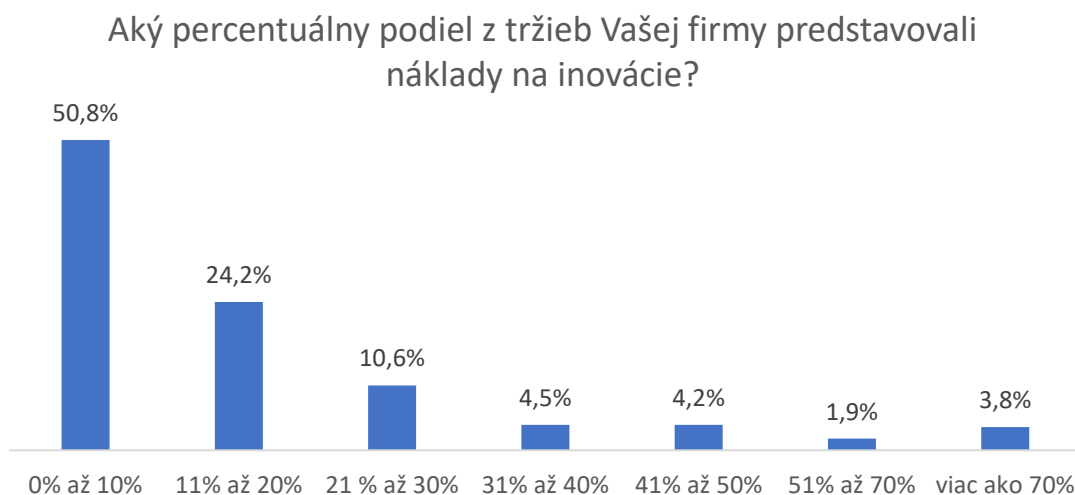
Graf č.32: Náklady na inovácie
